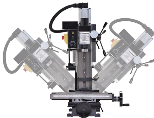
左右 45°傾斜可能
